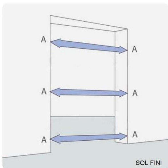
Réservation Largeur
