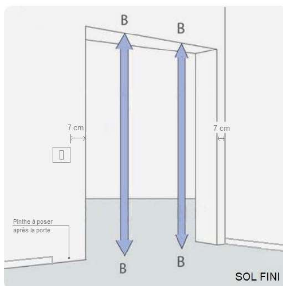
Réservation hauteur
